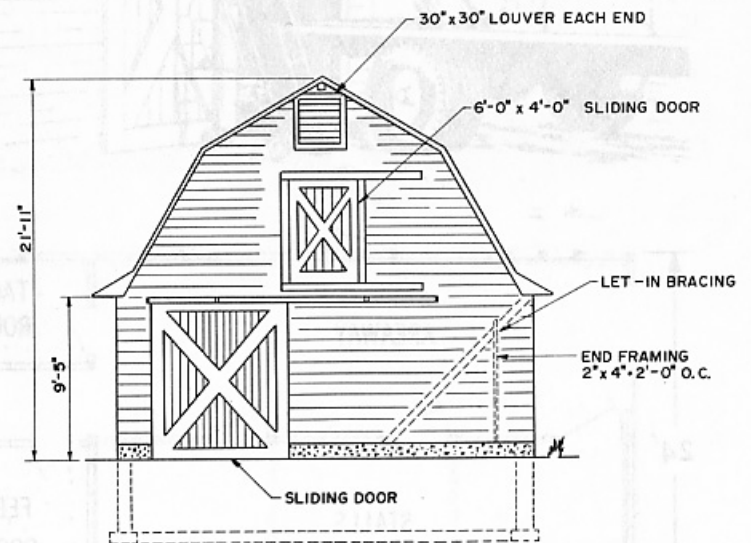
END ELEVATION
